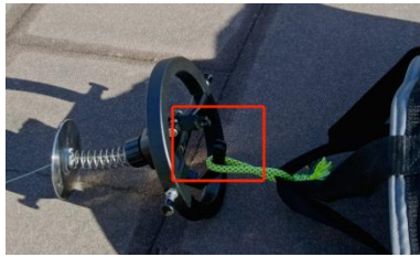
图 7-1-6 货物挂载于脱钩器凹槽处
