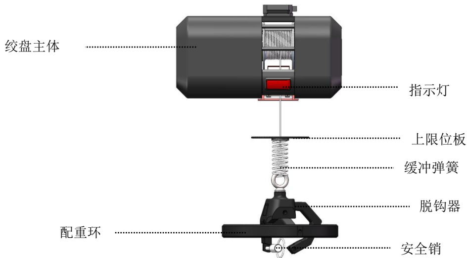
图 3-2-1 EayLoad-15 空载绞盘示意图 1
