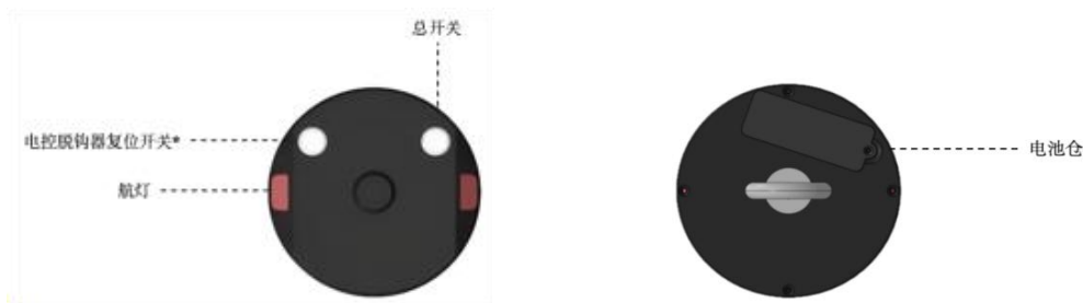
图 3-2-5 智能投放模块示意图
