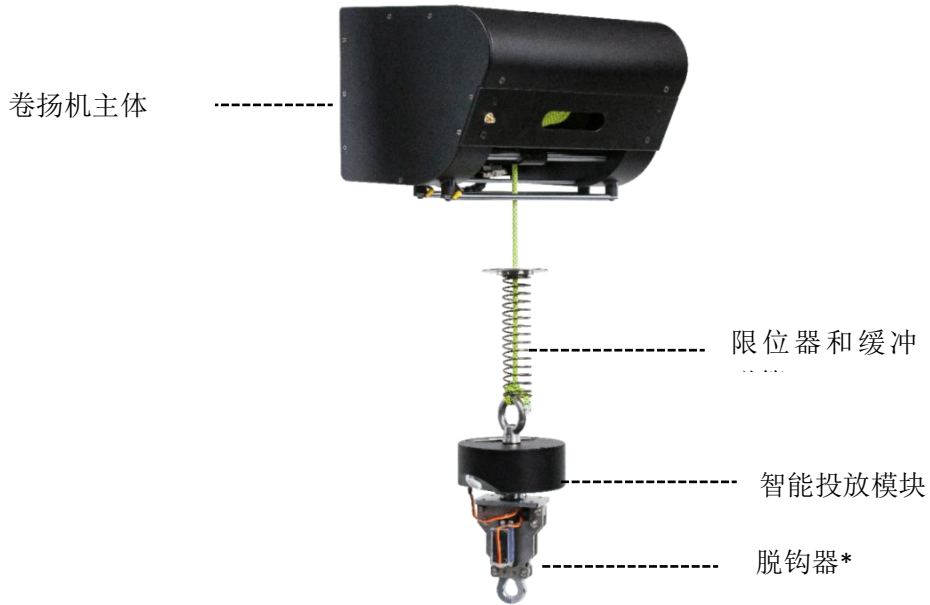
图 3-2-1 EayLoad-300 电动卷扬机示意图
